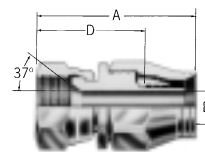
SAE 37° (JIC) swivel 63-190535-
