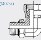
6901-NWO MAORB-FPS 90°
