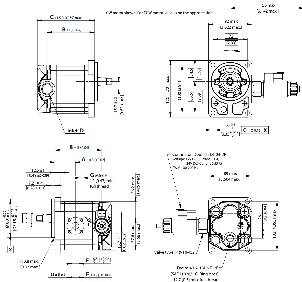
SGM2YN - 02AA dimensions
