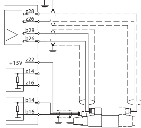
Amplifier models: 561, 568
