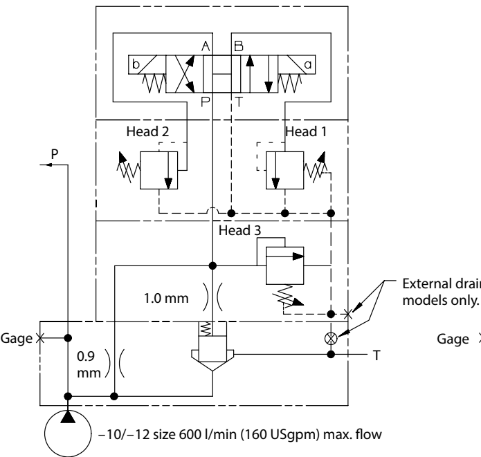
CPF3S-10/12-*-20 CPF3V-12-*-20
