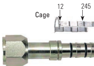
Cage groove
