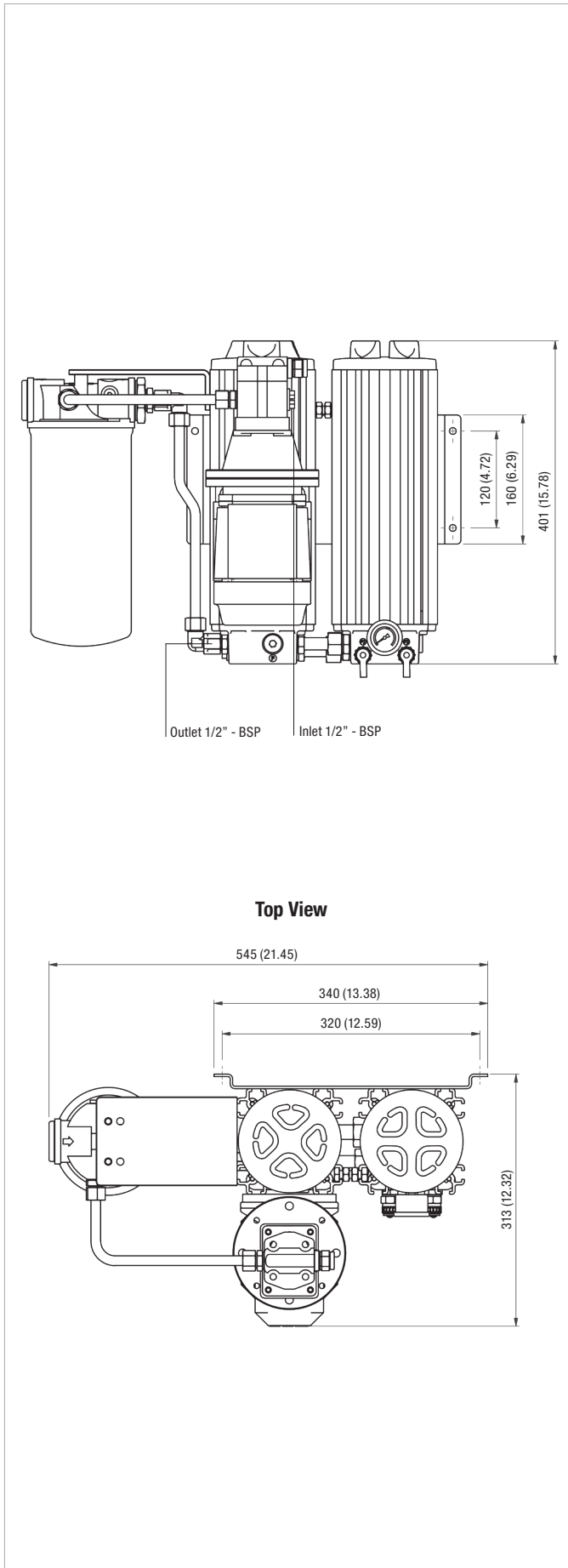
Dimensions OLSW-2-30
