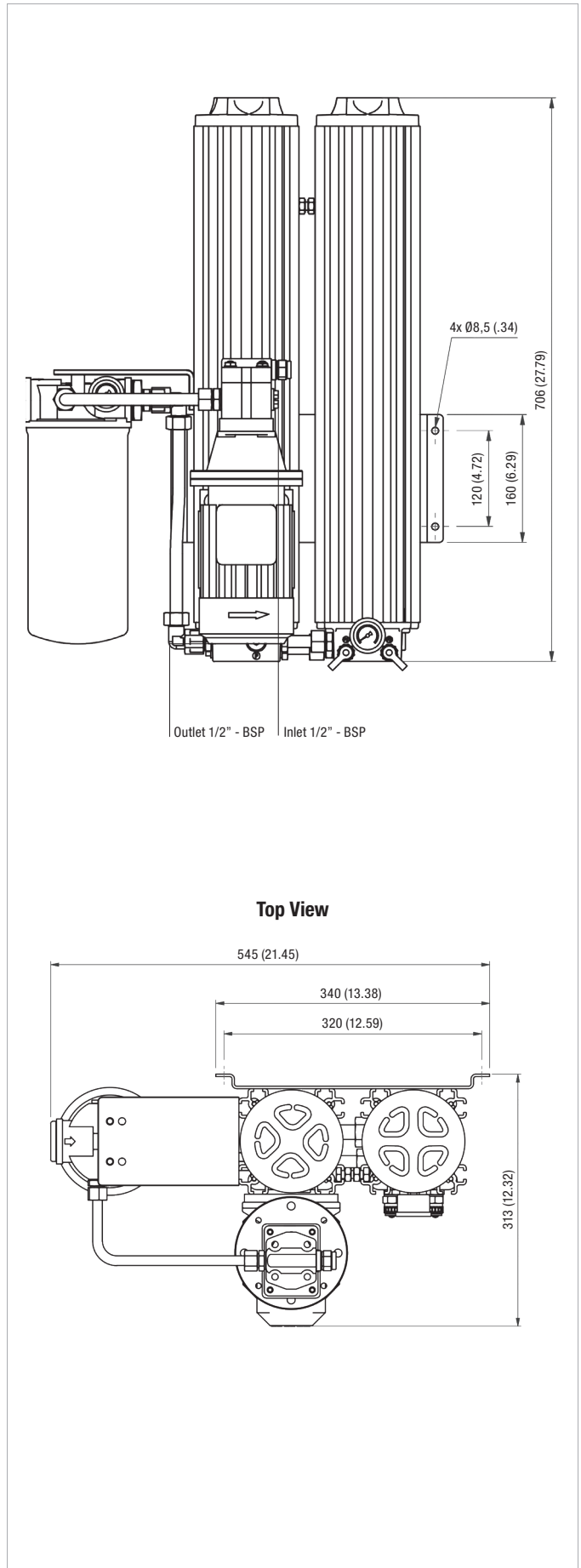
Dimensions OLSW-2-60
